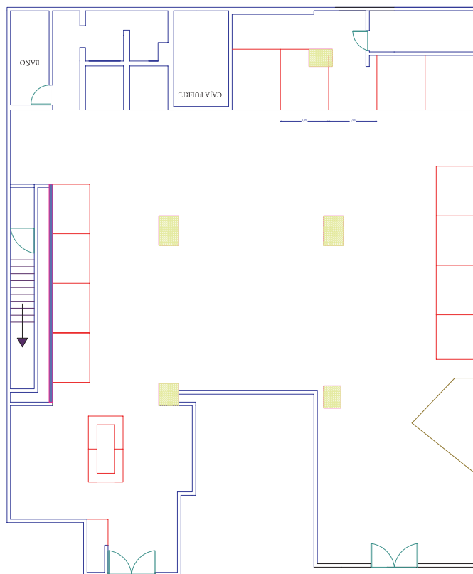
PLANTA DE PRIMER PISO PROPUESTA DE ADECUACION
