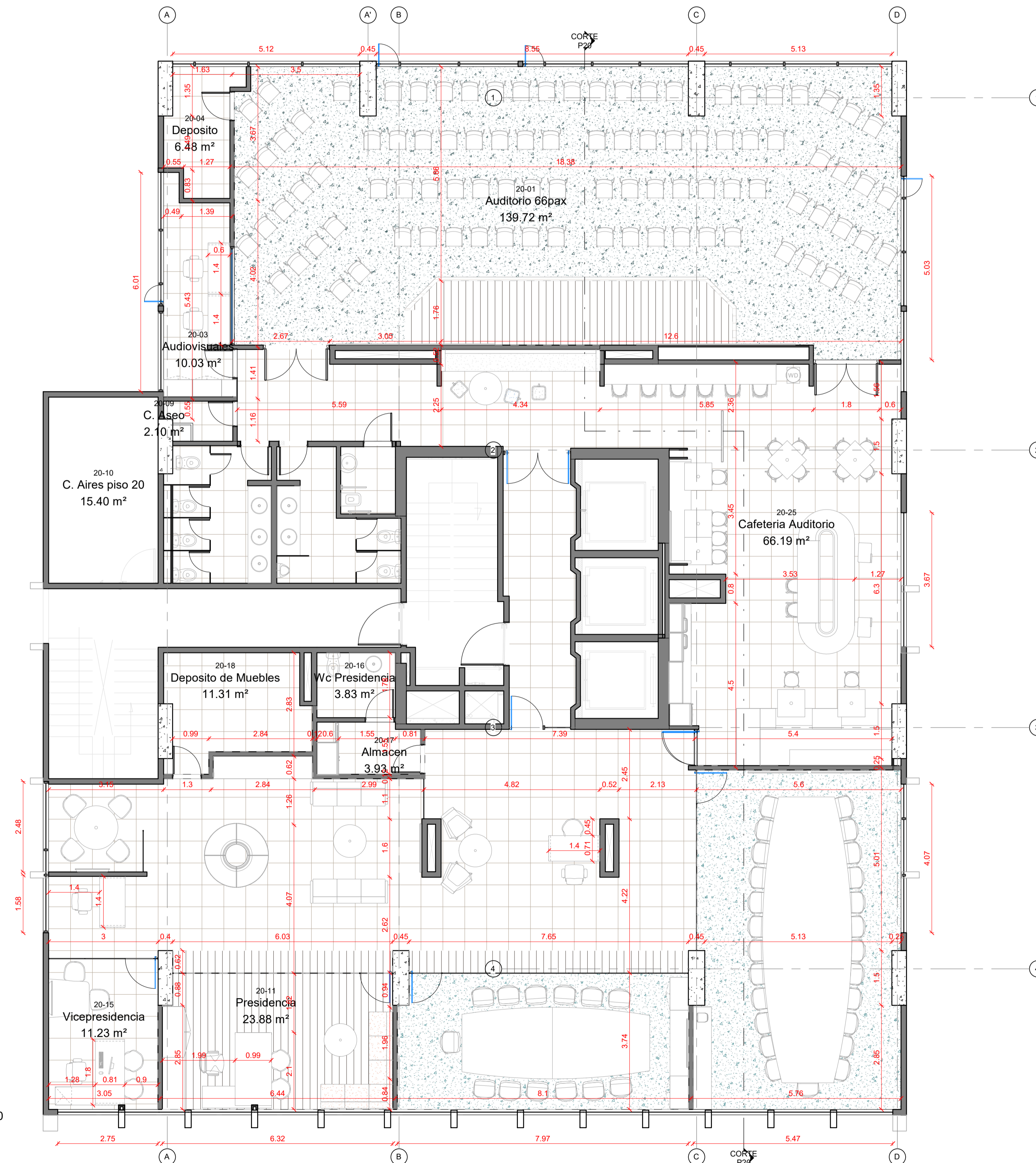
Arquitectura Piso 20 Escala 1:75
