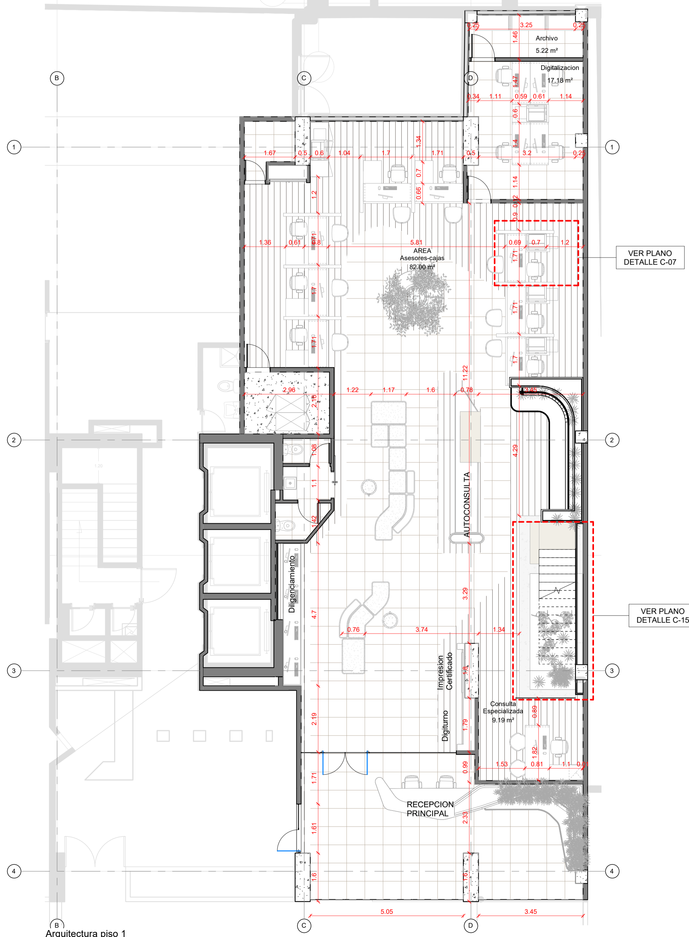
Arquitectura piso 1 Escala 1:75
