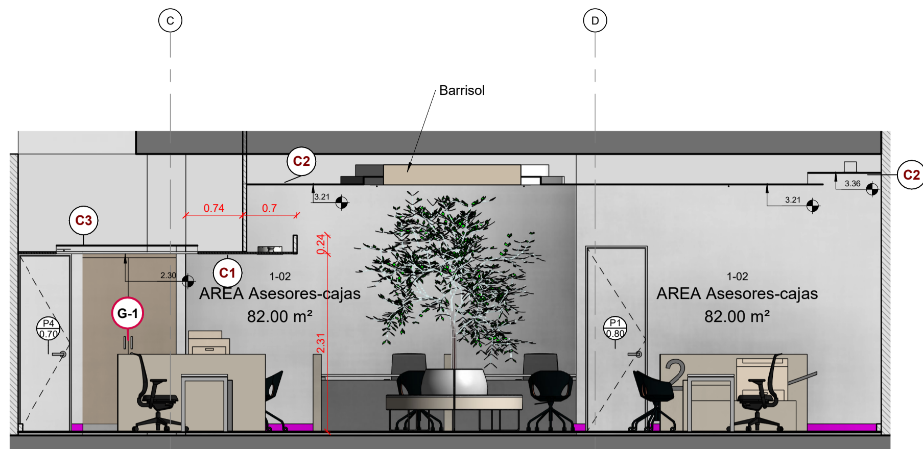
CORTE 1 - P1 Escala 1:50
