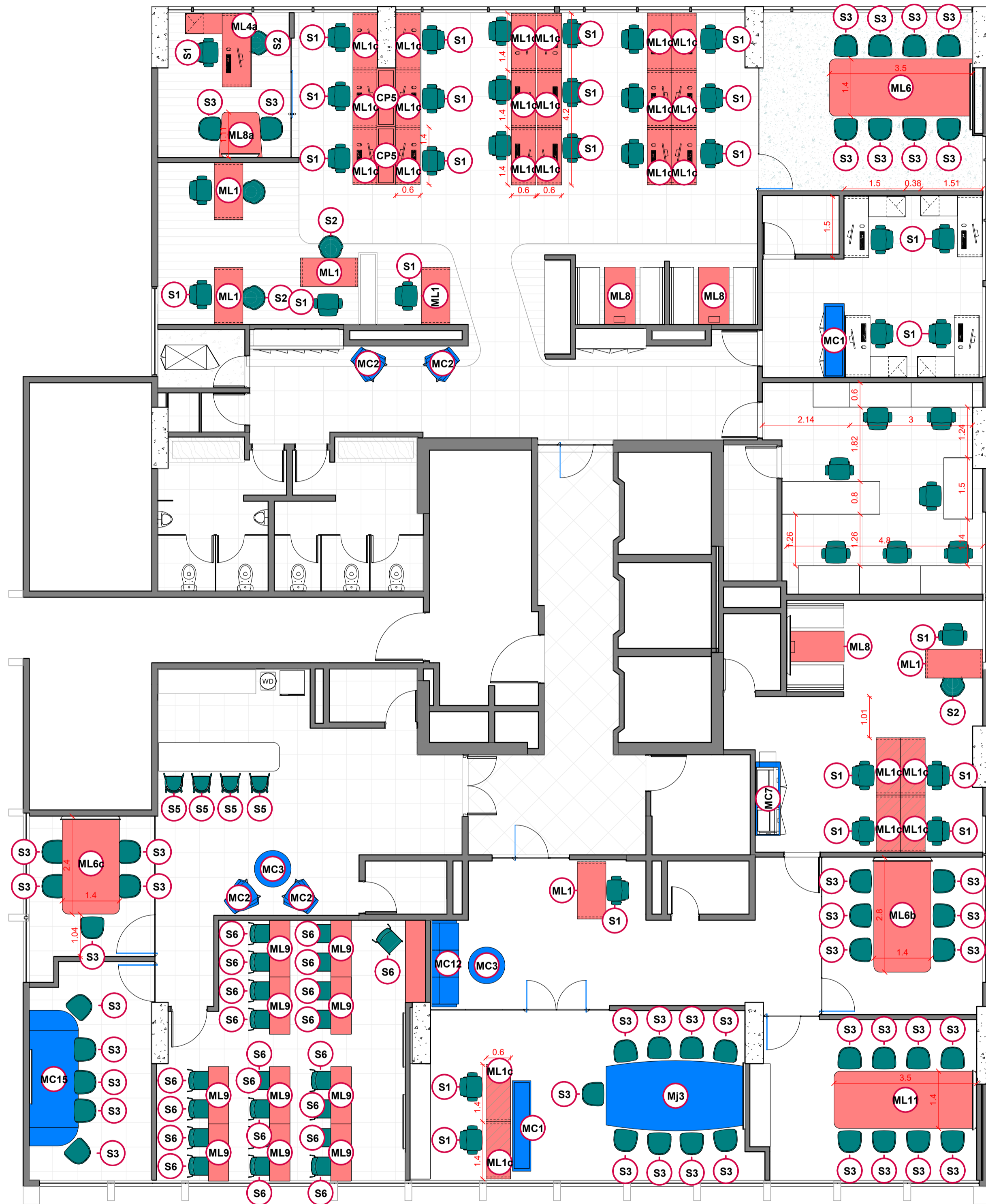
Mobiliario de Línea Piso 18 Escala 1 : 75
