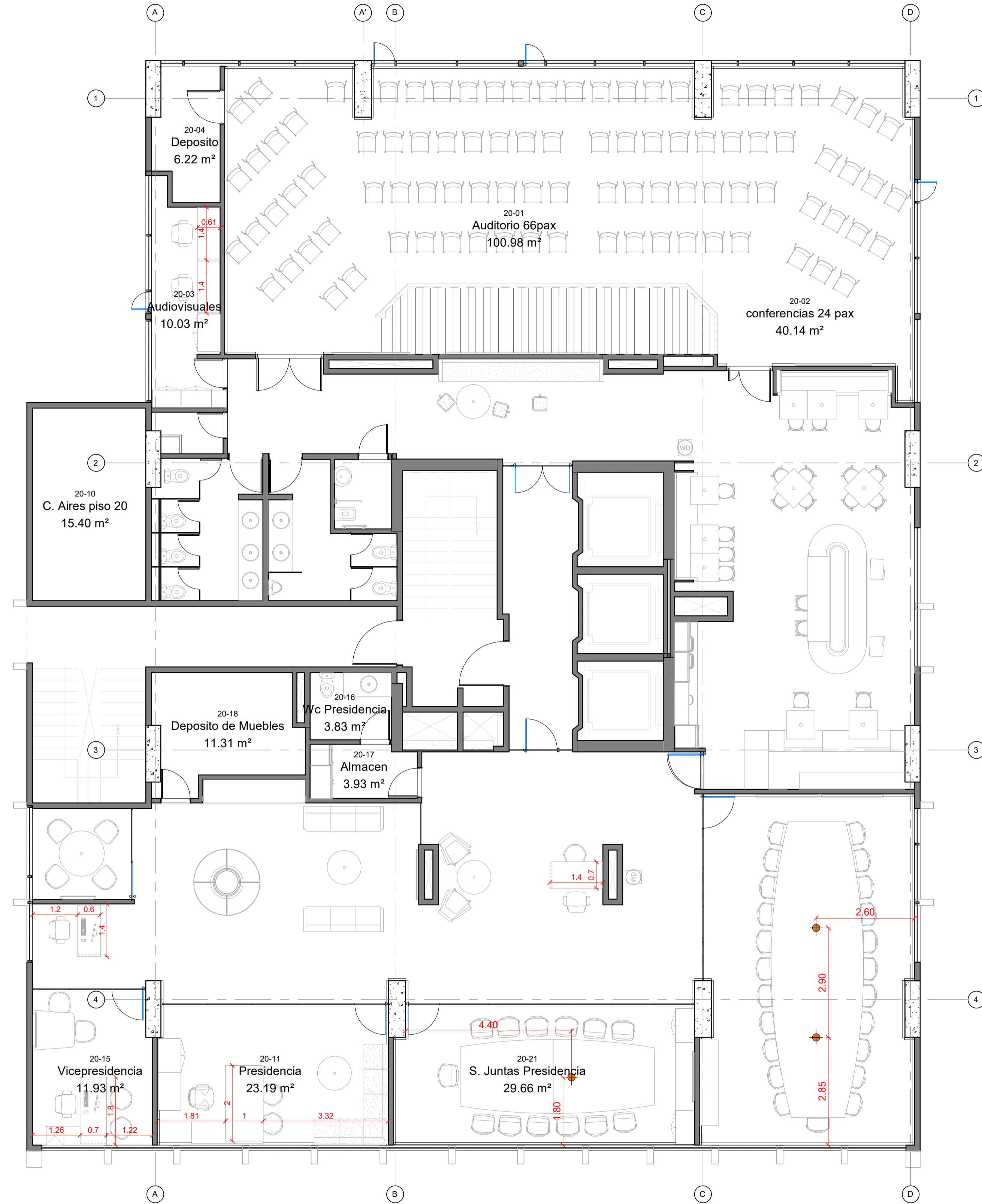
TOMAS EN PISO - P20 Escala 1 : 75
