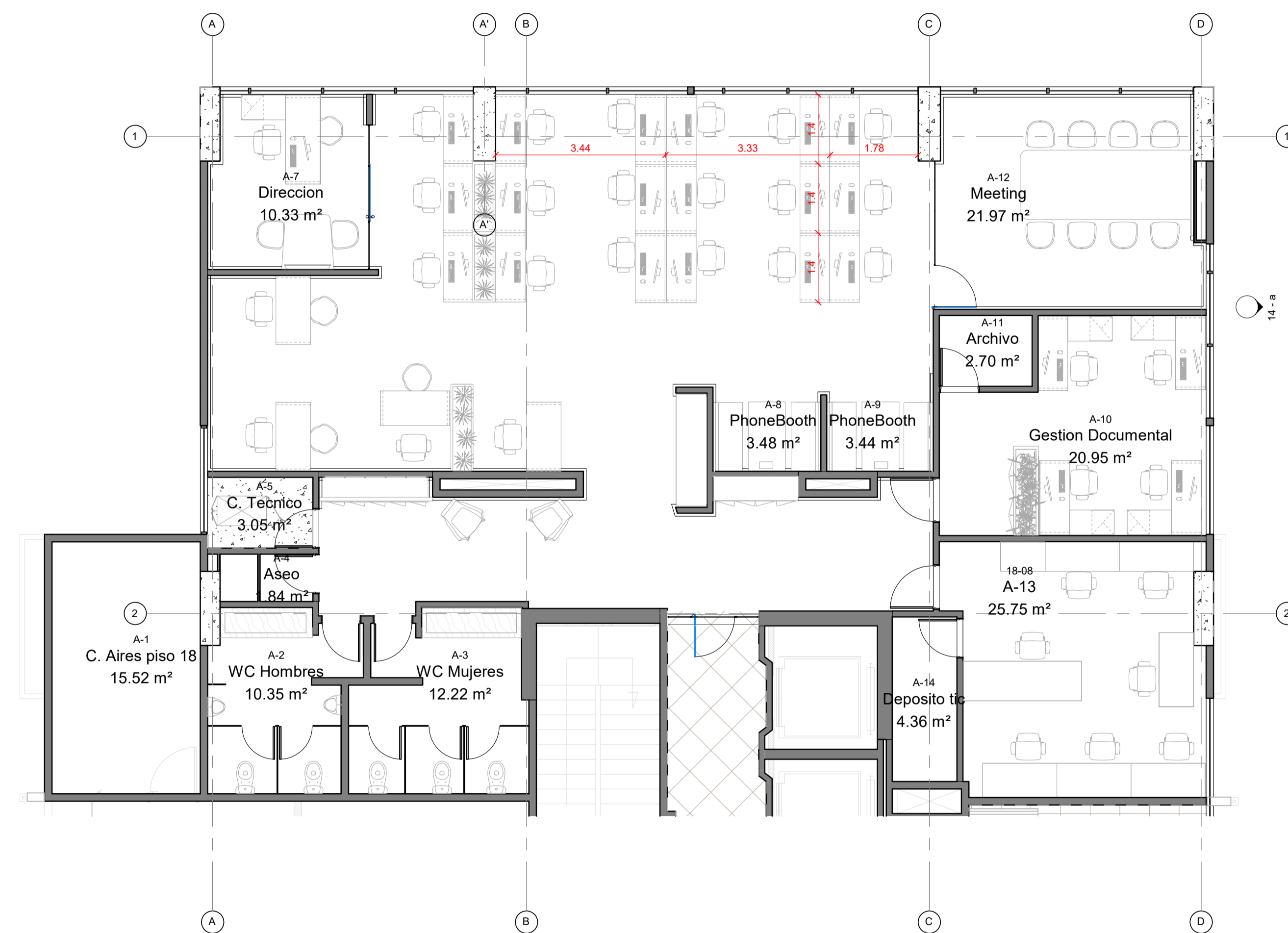
TOMAS EN PISO P18 Escala 1 : 75
