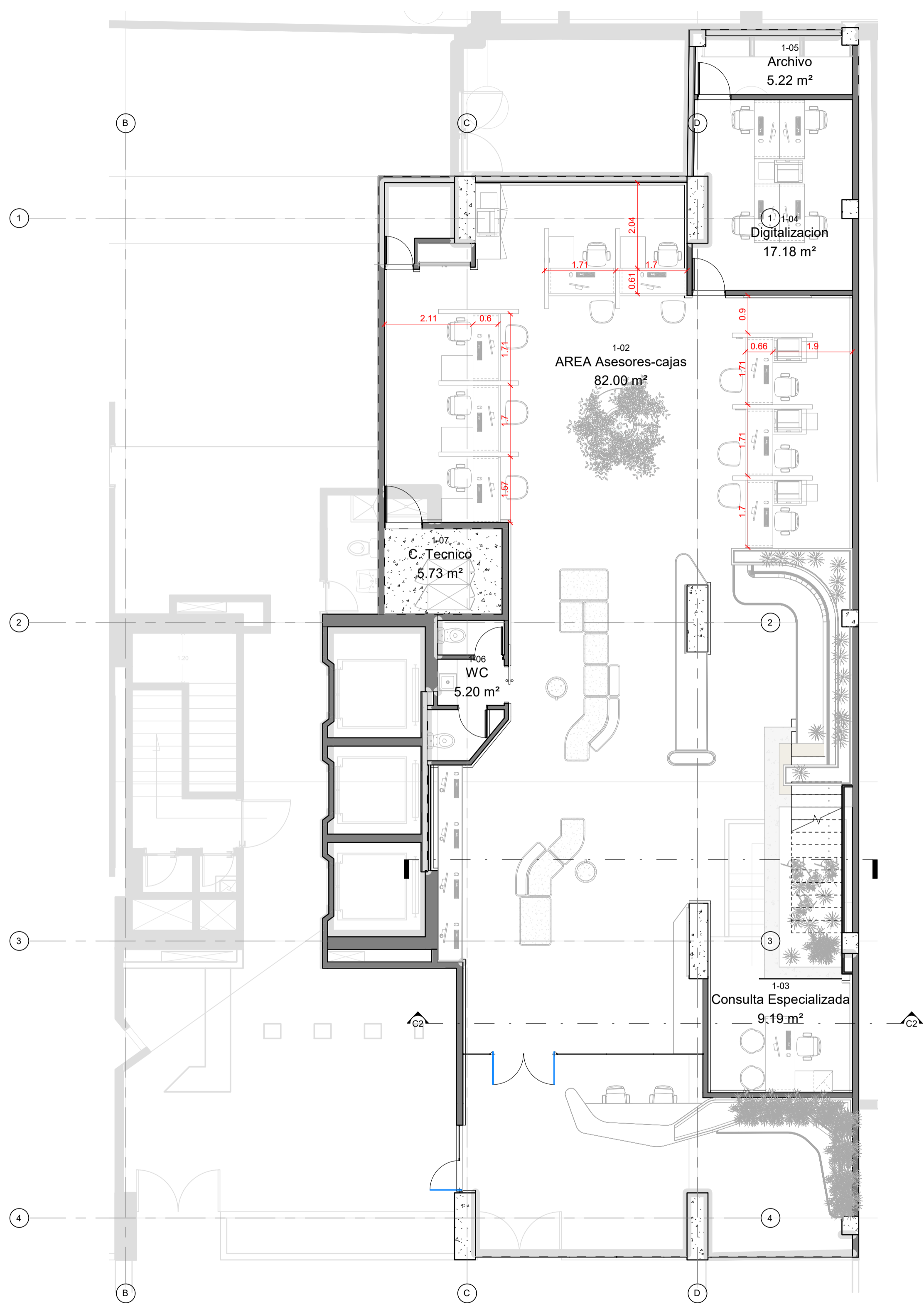
TOMAS EN PISO - P1 Escala 1:75
