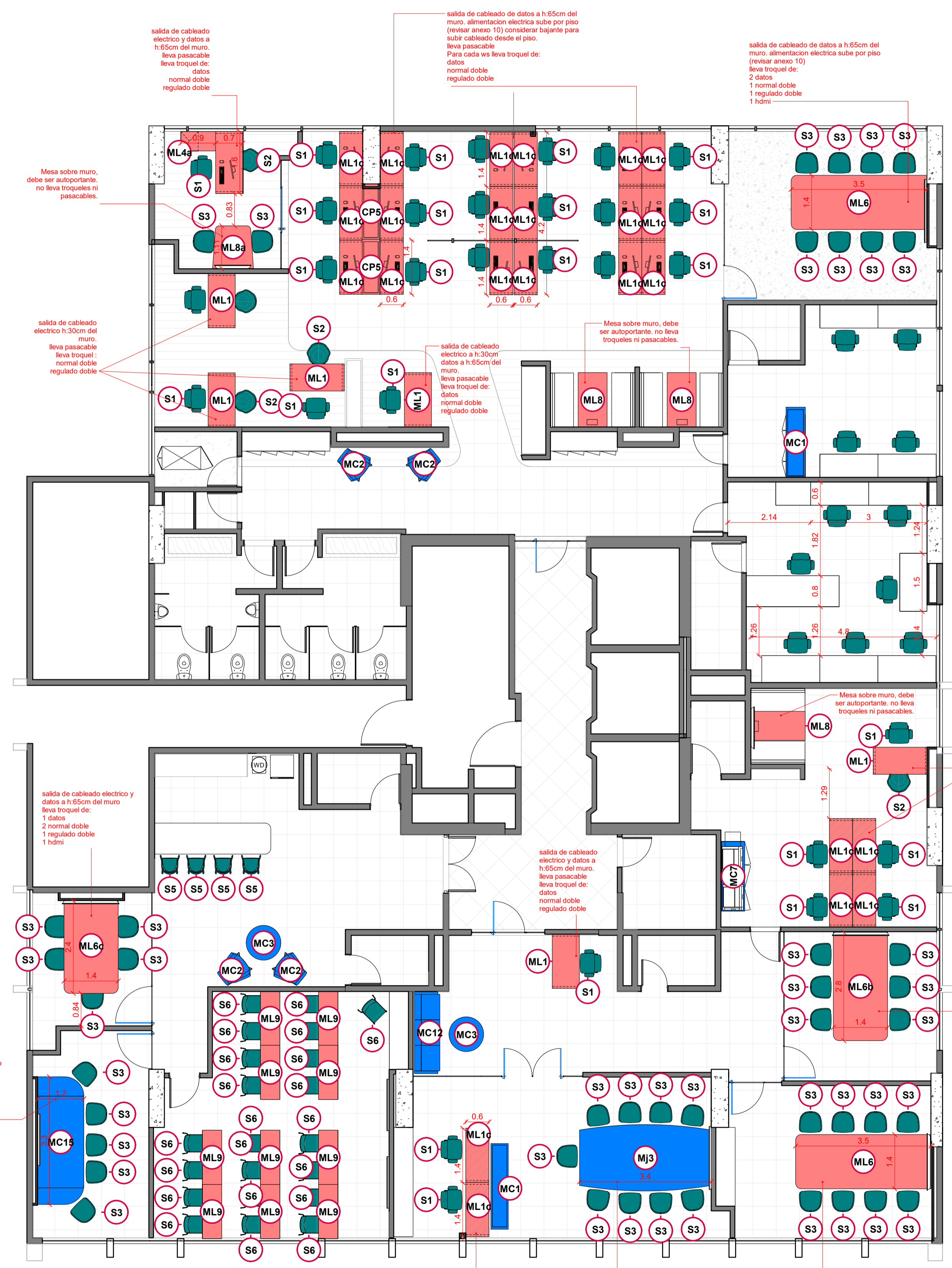
Mobiliario de Línea Piso 18 Escala: 1:75
