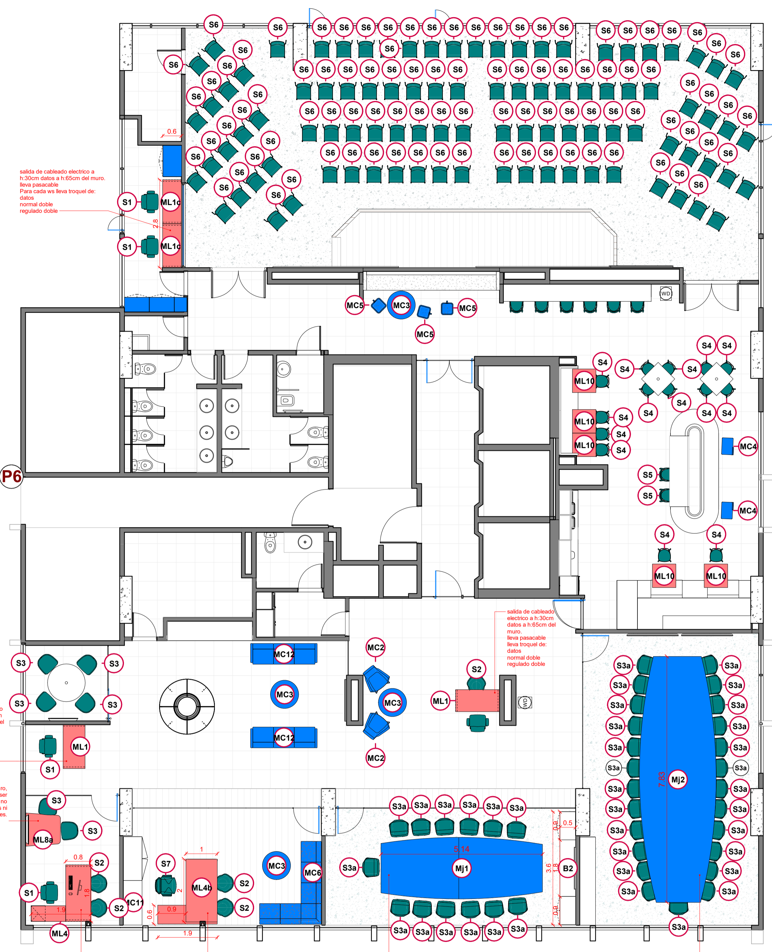
Mobiliario de Línea Piso 20 Escala 1:75
